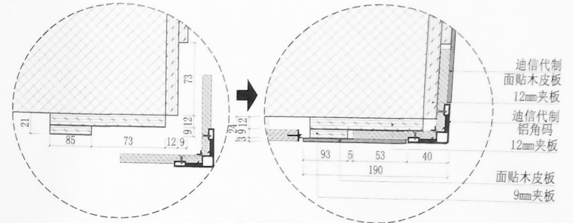
B 大样图
